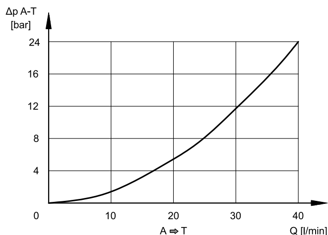
PRESSIONE MIN. REGOLATA p_{min} = f(Q)
