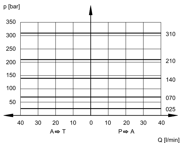
REGOLAZIONE p_{max} = f(Q)
