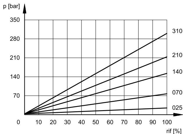
CONTROLLO PRESSIONE p = f(I)
