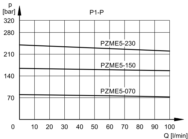
VARIAZIONE PRESSIONE p=f(Q)
