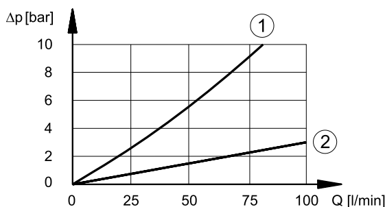
DRUCKVERLUSTE \Delta p = f(Q)
